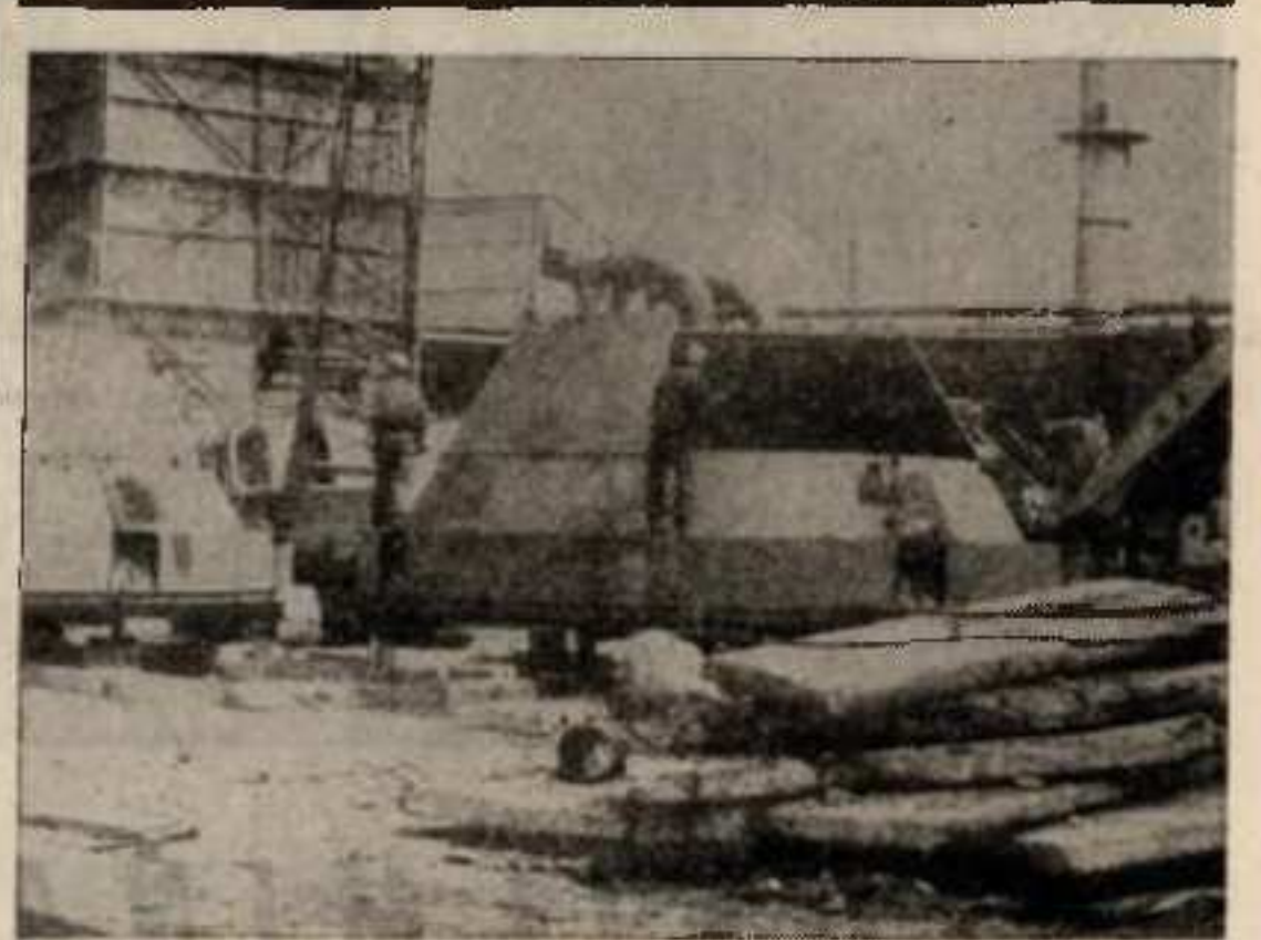
Wokół wielkiego pieca nr 1 rozpoczęto już prace przygotowawcze do remontu. Brygady z Huty Katowice przygotowują niezbędne elementy konstrukcyjne...
